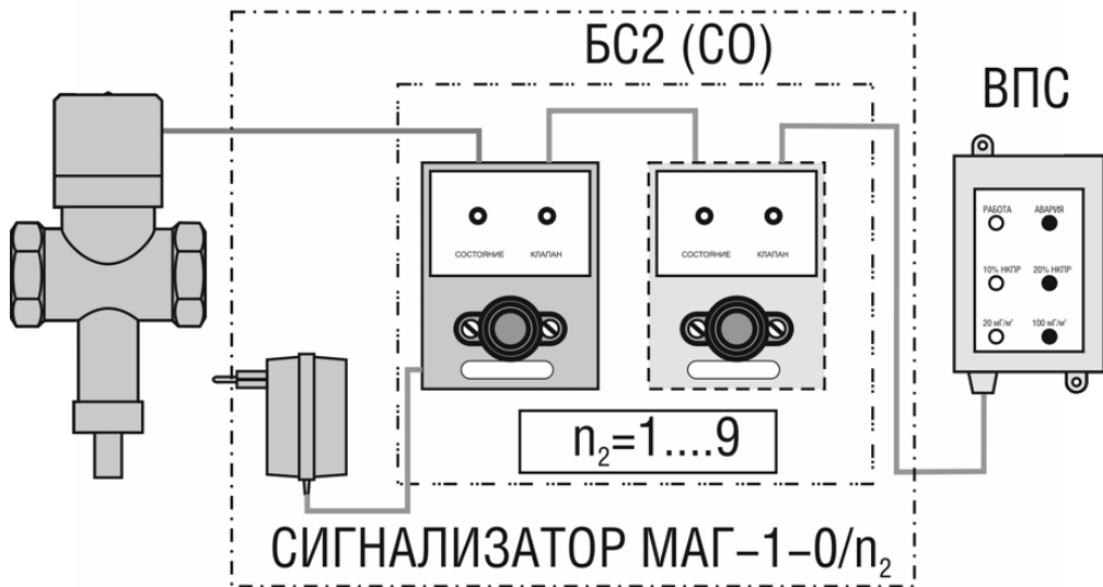
Фото ККЗ на базе МАГ1-01 и клапана КЗМЭМ
